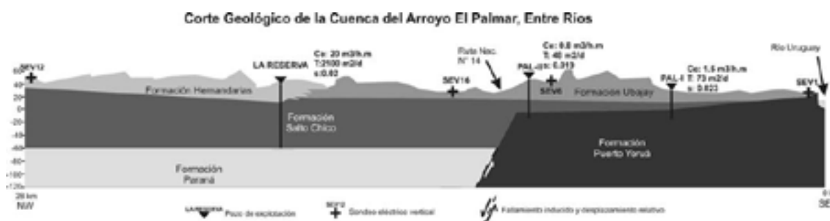
Figura 1. Modelo hidro-estratigráfico de la Cuenca del Arroyo El Palmar. Extraída de Busso y Machado, 2019.
